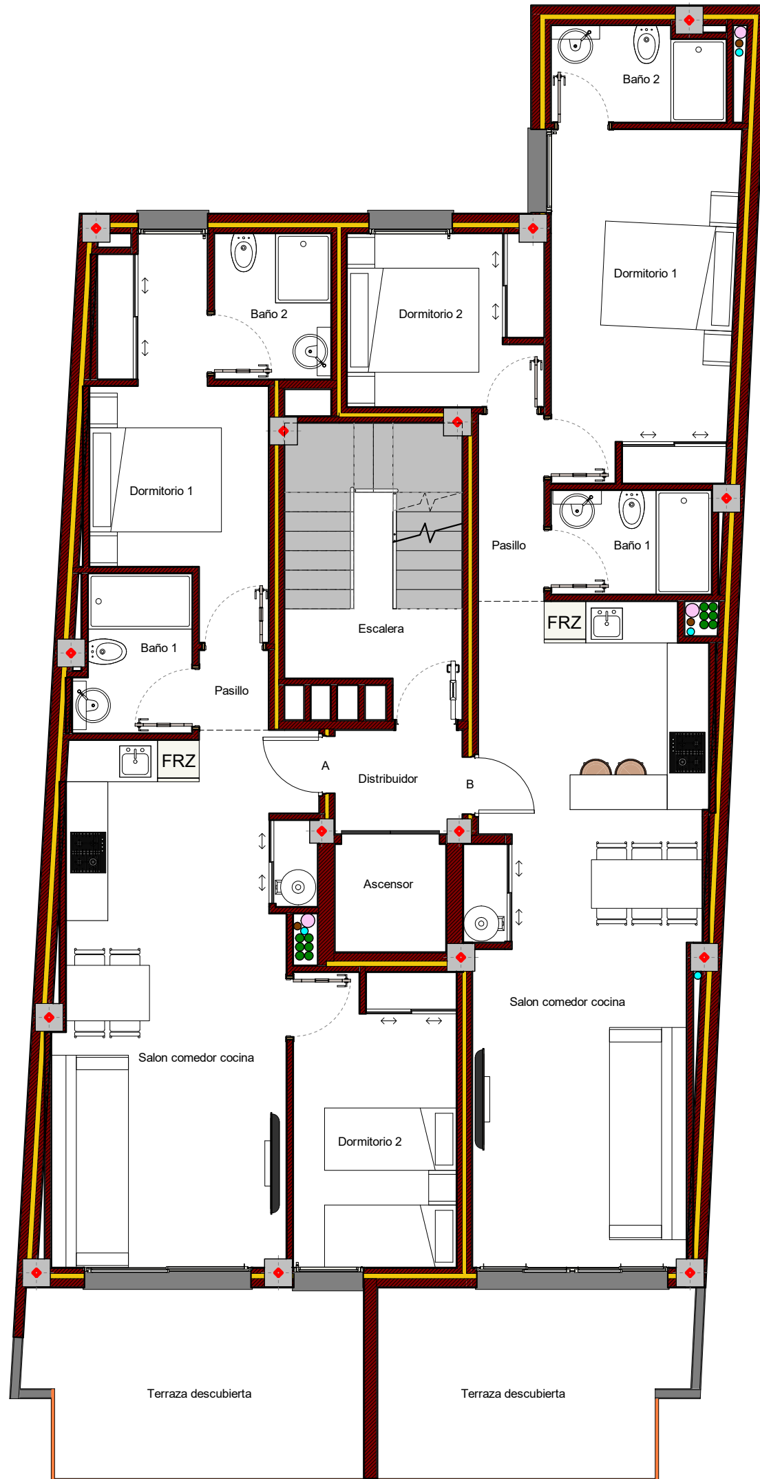
PLANTA ATICO CALLE RAMON GALLUD
